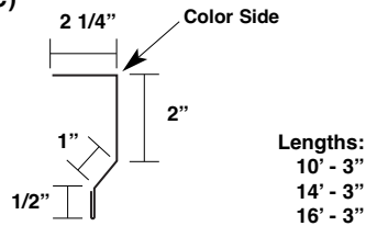
Overhead Door Drip 6 1/2" (P-ODP-6 1/2)
