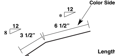
Gambrel Upper* (P-GU)
