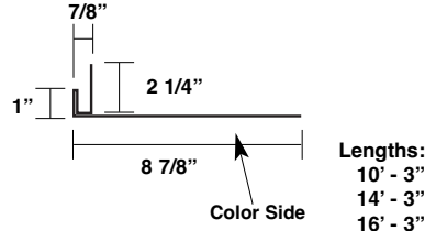
Corner Siding Door Jamb 6" (P-CSD-6)
