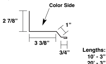
Ridge Trim* (R-RF)
