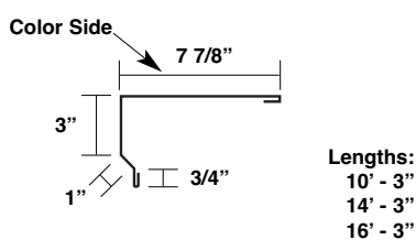
Overhead Door Flashing-A (P-JF-A)
