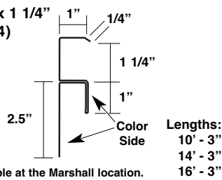
Door & Edge Cap (P-DEC)
