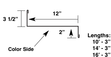
Valley Trim* (P-VF)
